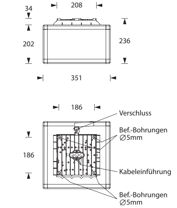
H-300 IP54 Gehäuseausführung / Casing design / Configuration logement 351 x 236 x 351 mm
